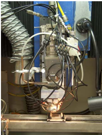
Optique de rechargement-fabrication directe par injection coaxiale de poudres
